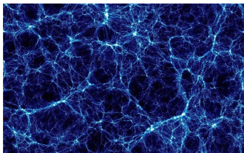
Космическая паутина Вселенной.
